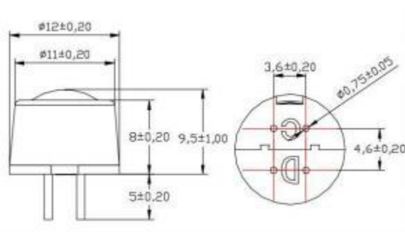
图 1： 传感器外形结构
