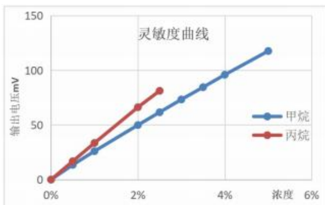
图 3：灵敏度曲线
