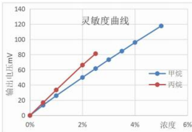
图 3: 灵敏度曲线
